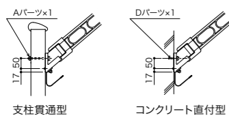
支柱貫通型
