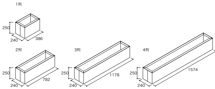
巾木サイズ
