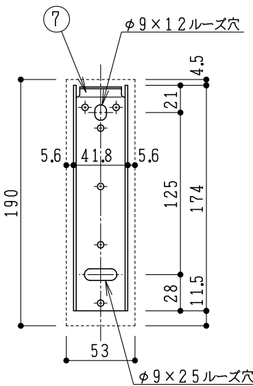
Eブラケット受 取付図 S=1/4
