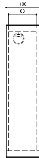
右開き取出側姿図
