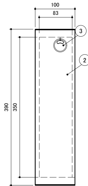
左開き取出側姿図
