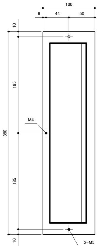
裏面図
