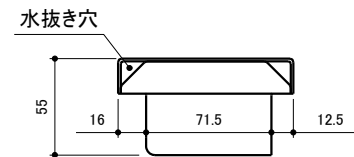
底面図
