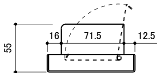
平面図
