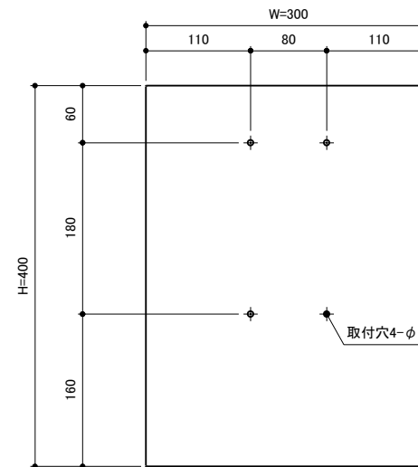
背面図
