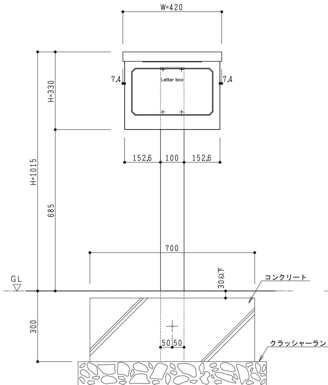
SWING用スタンド 姿図 S=1/10
