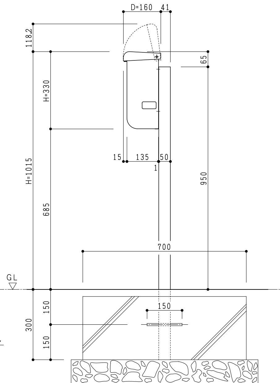
側面図 S=1/10
