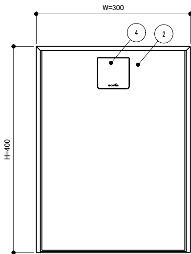
正面姿図
