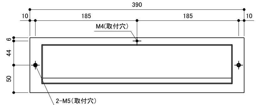
裏面図
