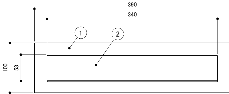
正面図
