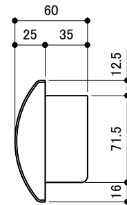
側面図
