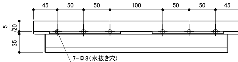
底面図
