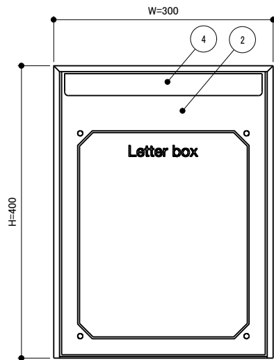
正面図
