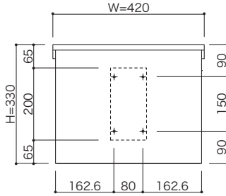
アンカーポイント図
